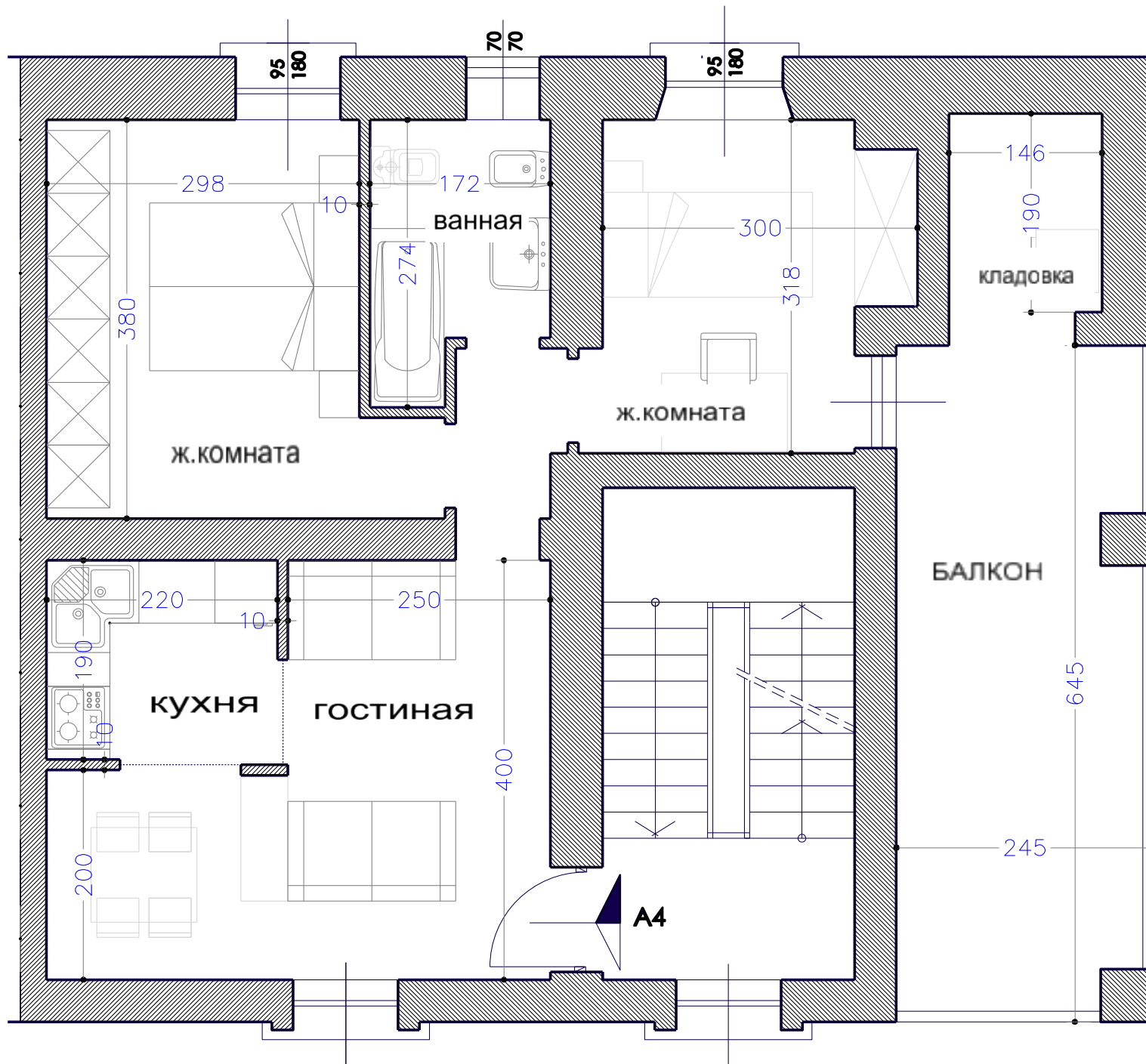
ВТОРОЙ ЭТАЖ
